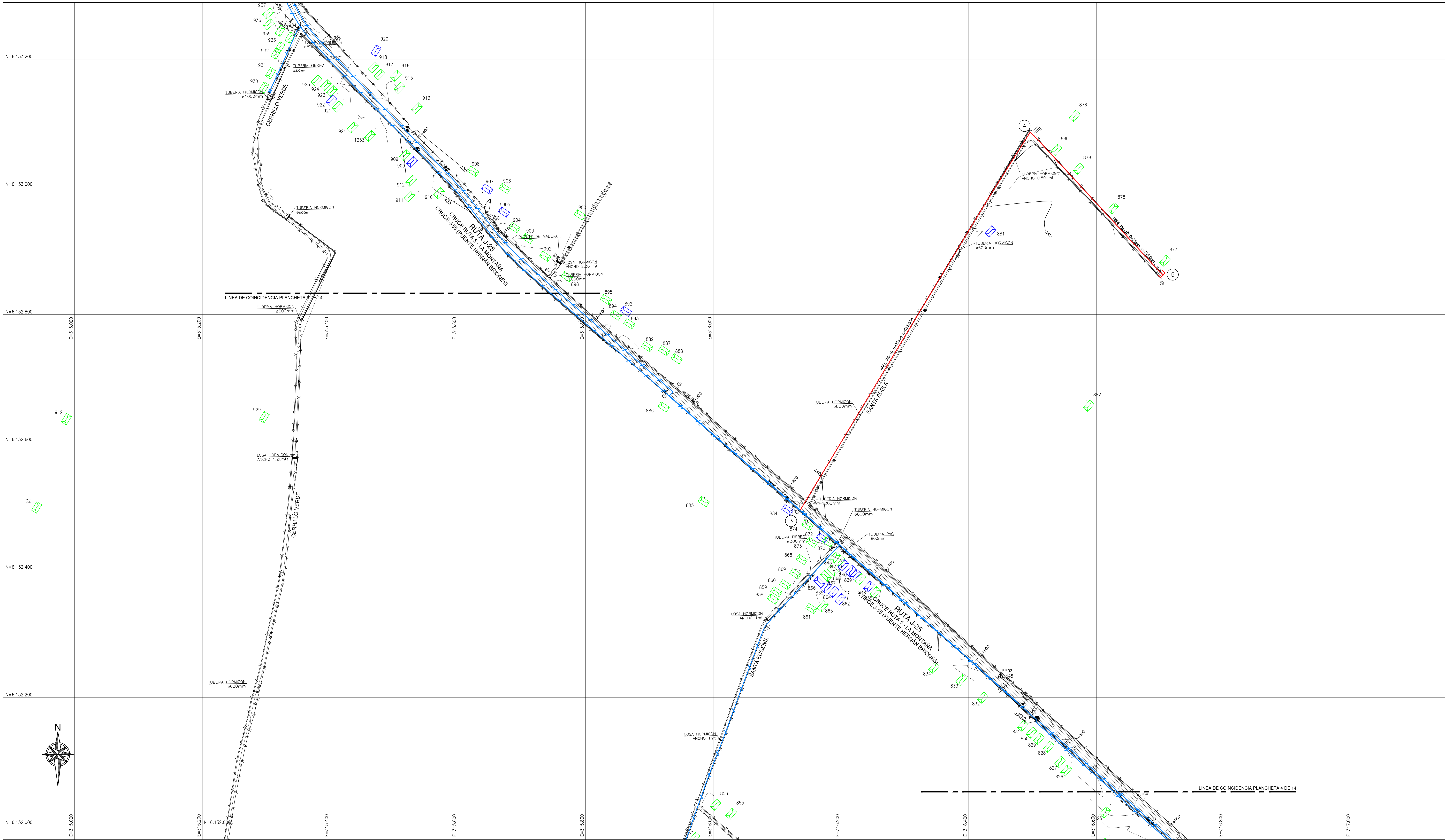
PLANTA RED PROYECTADA PLANCHETA 3 DE 14 ESCALA 1 : 2.000
